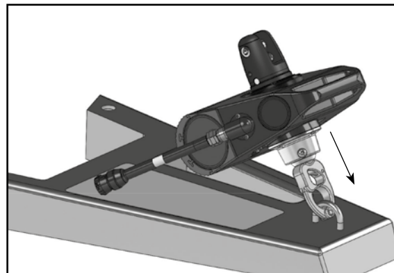
Fixer le motoréducteur sur point d'ancrage prévu. Install the gear motor on the fastening point
